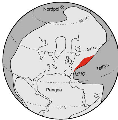
Spätes Perm (ca. 250 MioJ)
