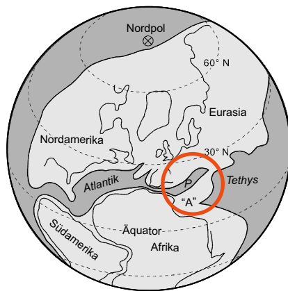
Später Jura (ca. 140 MioJ)
